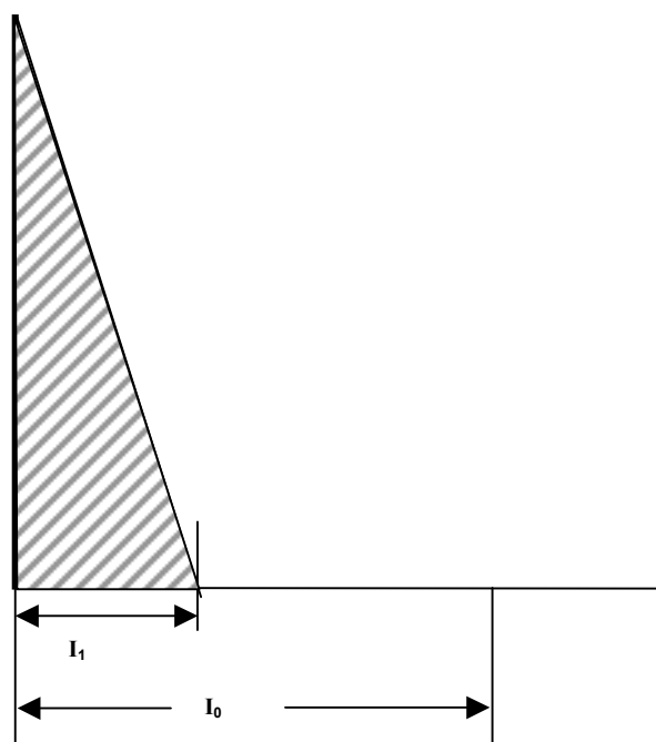
Рис.2А. График распределения тока вдоль антенны. Ненастроенный укороченный штырь. Длина штыря h=2,4 м., частота F=4,0 МГц. Антенна не настроена в резонанс. Согласование производится с помощью антенного тюнера. I_0 – Максимальный ток на выходе антенного тюнера, или ток на входе четверть волнового штыря I_1 – максимальный ток на входе укороченной антенны.
